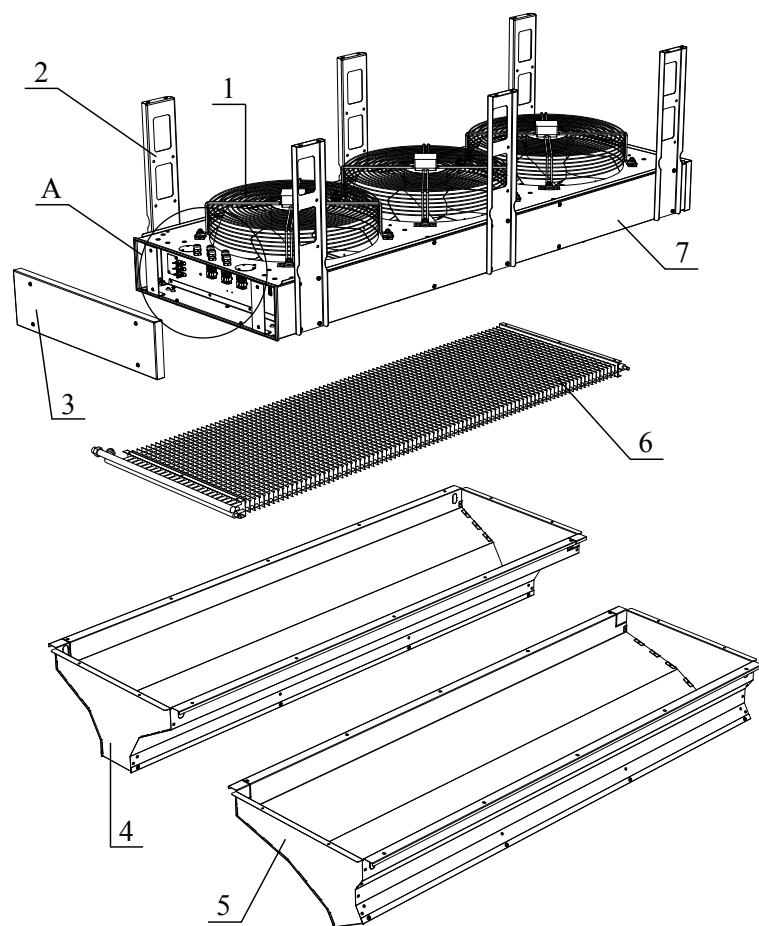
Рисунок 2. Воздушно-тепловая завеса
