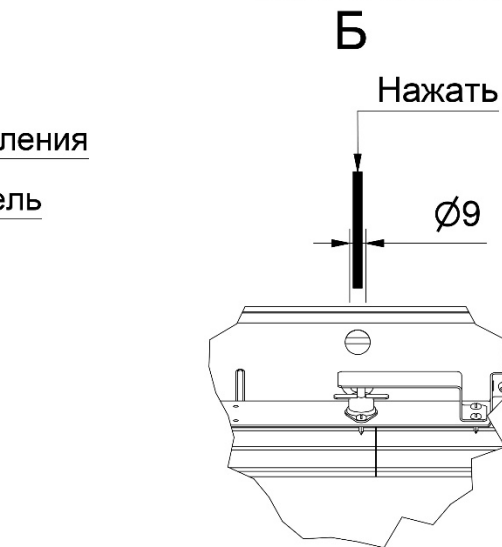
Рисунок 4-Аварийный термовыключатель
