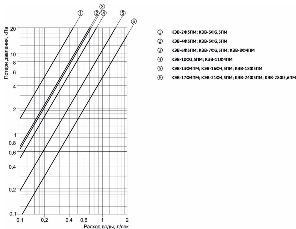
Рисунок 7 – Гидравлические характеристики
