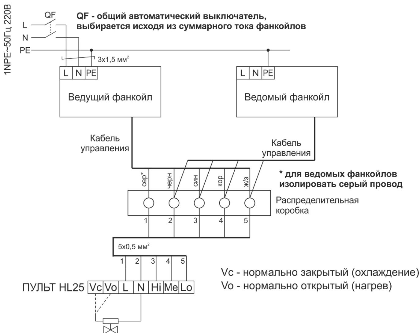
Рисунок 3 - Групповое подключение фанкойлов одной модели к пультау HL25
