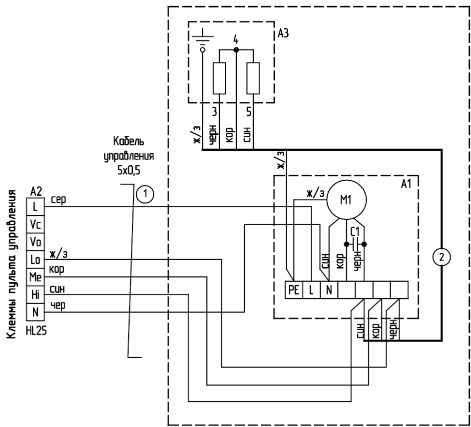
Рисунок 8 – Схема электрическая КЭВ-3Ф3ПМ, КЭВ-14Ф4,5ПМ, КЭВ-19Ф4,5ПМ
