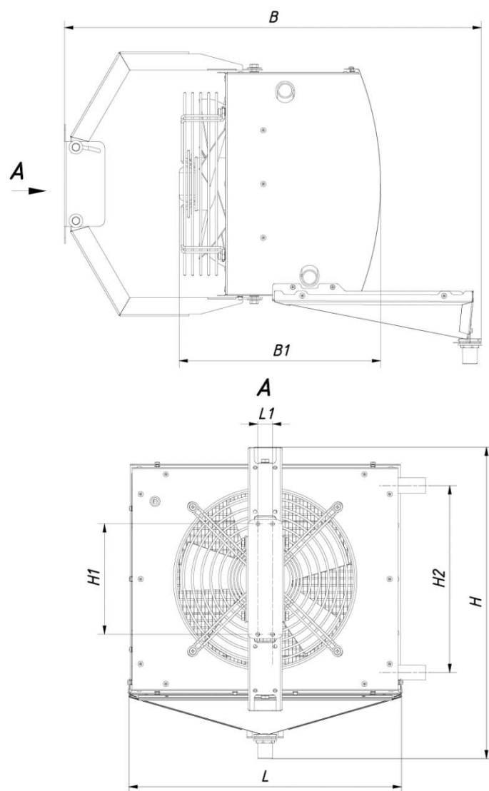
Рисунок 6 – Габаритные и присоединительные размеры
